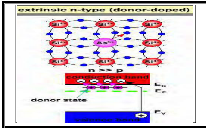
الشكل (9-2) يبين شبه موصل نوع (n-type) [63].
