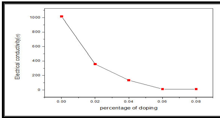
الشكل (28-4) التوصيلية الكهربائية كدالة لنسب التطعيم لاغشية (CdO) غير المطعمة
