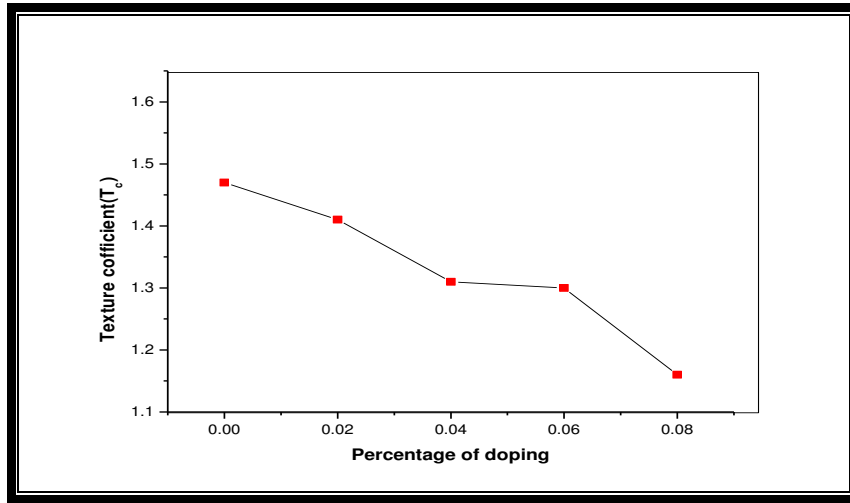
الشكل (3-4) قيم عامل التشكيل كدالة لنسب التطعيم.
