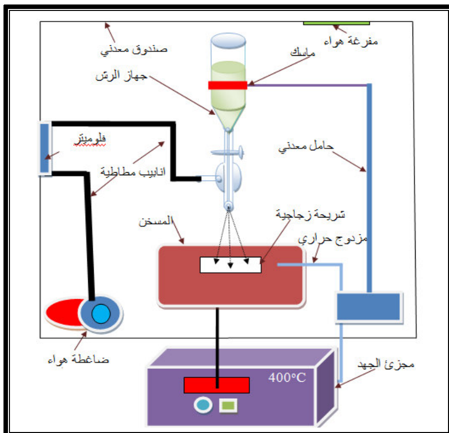
الشكل (2-3) منظومة التحلل الكيميائي الحراري
