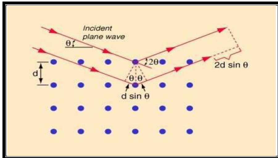
الشكل (11-2) المستويات البلورية لقانون براك [70] .
