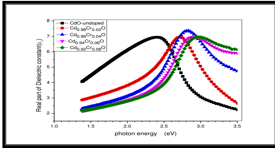
الشكل (23-4) تغير ثابت العزل الحقيقي كدالة لطاقة الفوتون لأغشية (CdO) غير المطعمة والمطعمة بالكروم.
