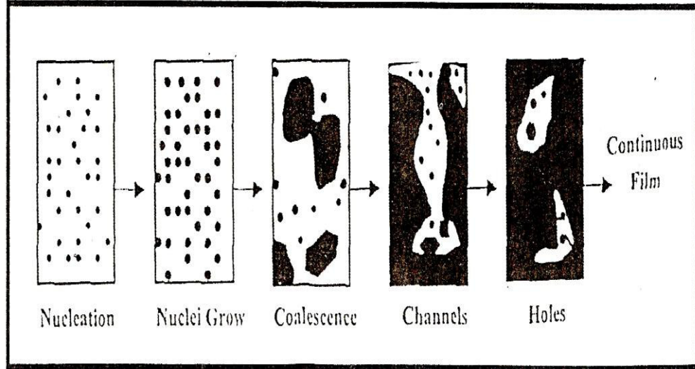
الشكل (2-1) المراحل الاساسية لتكوين الأغشية الرقيقة [9].
