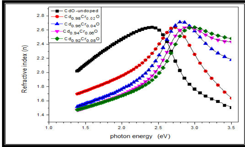
الشكل (4-19) تغير معامل الانكسار كدالة لطاقة الفوتون لأغشية (CdO) غير المطعمة والمطعمة بالكروم.
