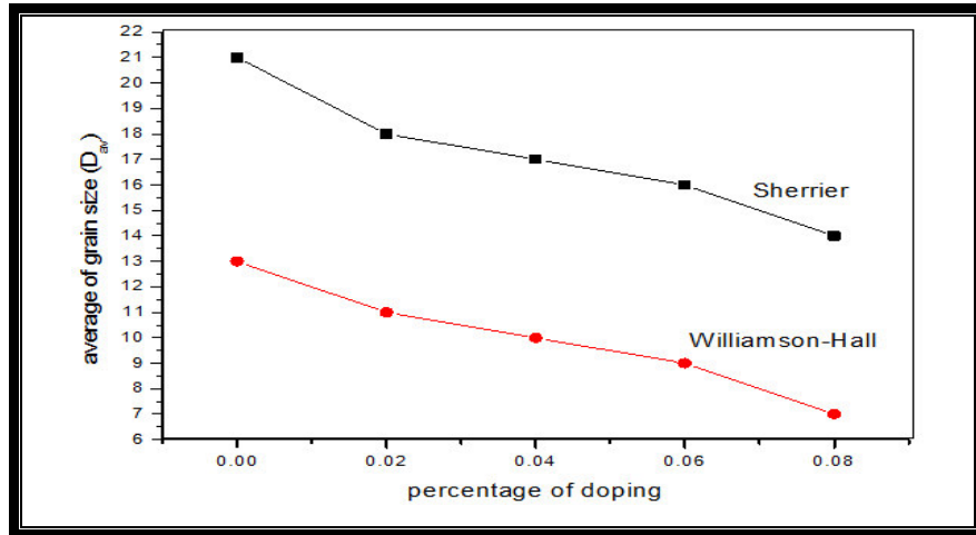
الشكل (2-4) قيم معدل الحجم الحبيبي كدالة لنسب التشويب.
