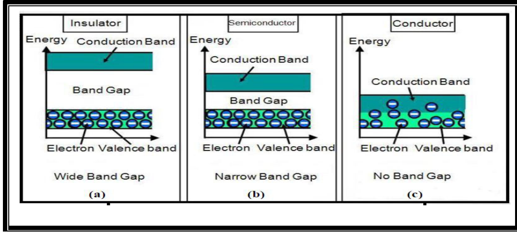
الشكل (7-2) حزم الطاقة في المواد ، (a-عازل)، (b - شبه موصل)، (c - موصل) [57].
