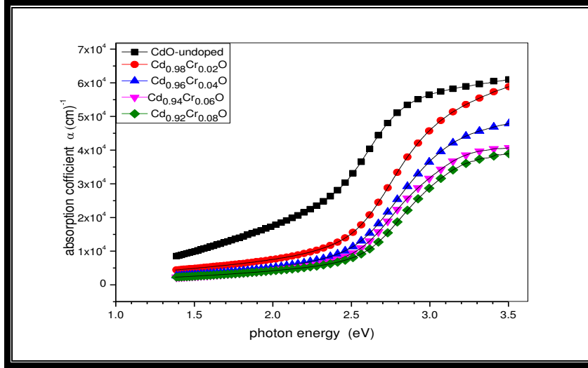
الشكل (10-4) تغير معامل الامتصاص مع طاقة الفوتون لاغشية (CdO) غير المطعمة والمطعمة بالكروم.
