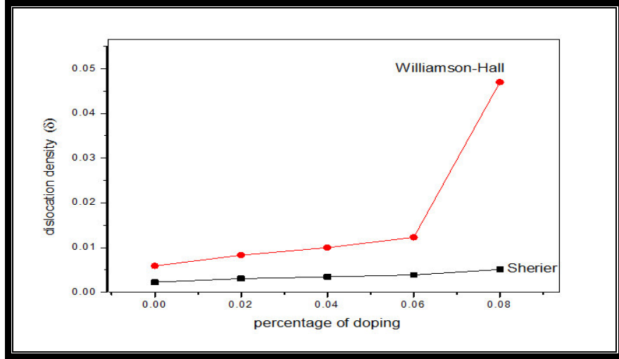
الشكل (4-4) قيم كثافة الانخلاعات كدالة لنسب التطعيم.
