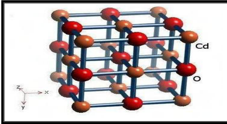
الشكل (4-1) التركيب البلوري لأوكسيد الكاديوم [14].
