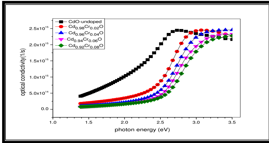
الشكل (4-25) العلاقة بين التوصيلية البصرية كدالة لطاقة الفوتون لاغشية (CdO) غير المطعمة والمطعمة بالكروم.
