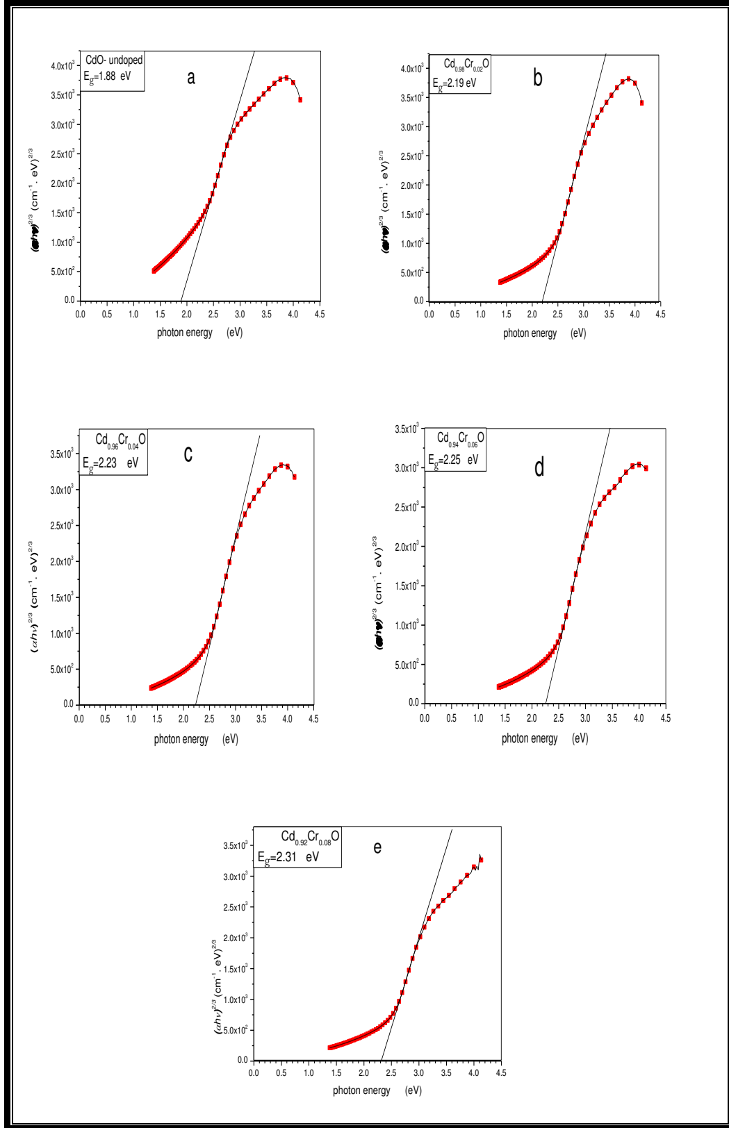
الشكل (14-4a,b,c,d,e) قيم فجوة الطاقة للانتقال المباشر الممنوع كدالة لطاقة الفوتون لاغشية (CdO) غير المطعمة والمطعمة بالكروم.
