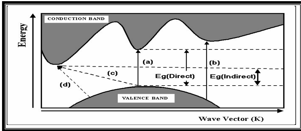
شكل (16-2) الانتقالات الالكترونية [93]
