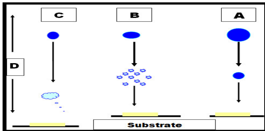
الشكل (3-1) حجم القطرات (A) كبيرة، (B) متوسطة (الحالة المثالية)، (C) صغيرة [10].
