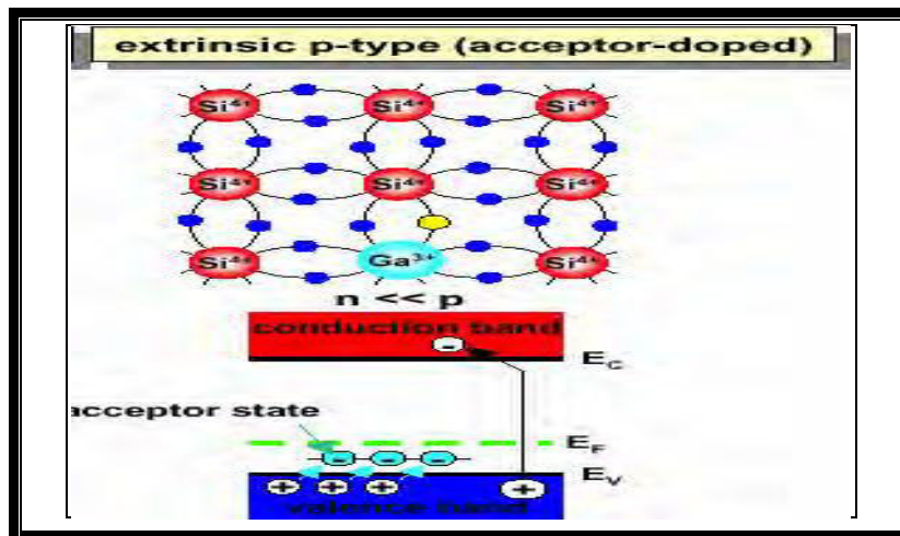
الشكل (10-2) يبين شبه موصل من النوع (p-type) [63].
