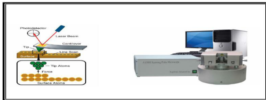
الشكل (3-4) يظهر مجهر القوة الذرية من النوع (AA 3000) مع مخطط لآلية عمله [74].
