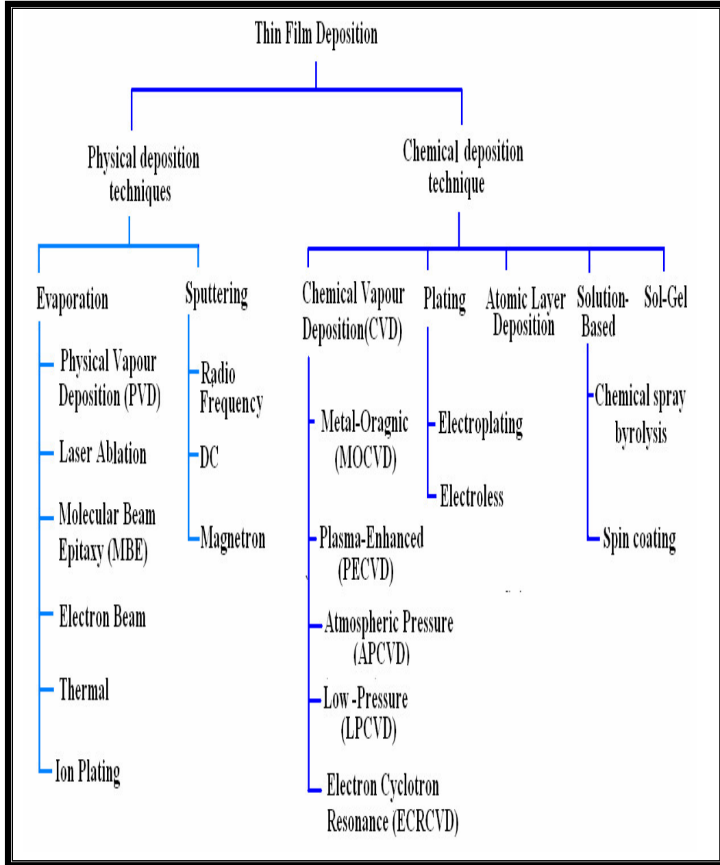
الشكل (1-1) طرائق تحضير الاغشية الرقيقة [7].
