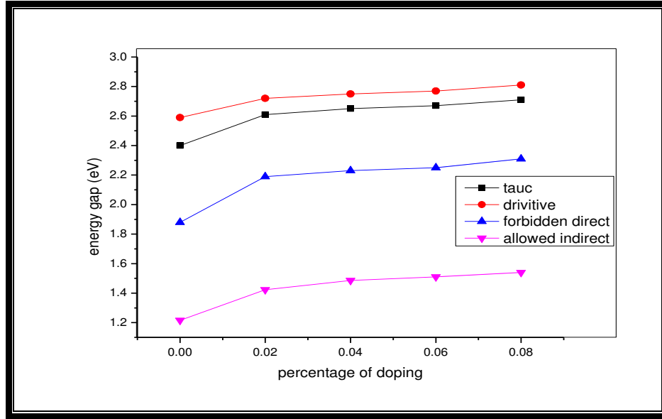
الشكل (4-13) تغير فجوة الطاقة البصرية للانتقالات الالكترونية المحسوبة كدوال لنسب التطعيم لأغشية (CdO).
