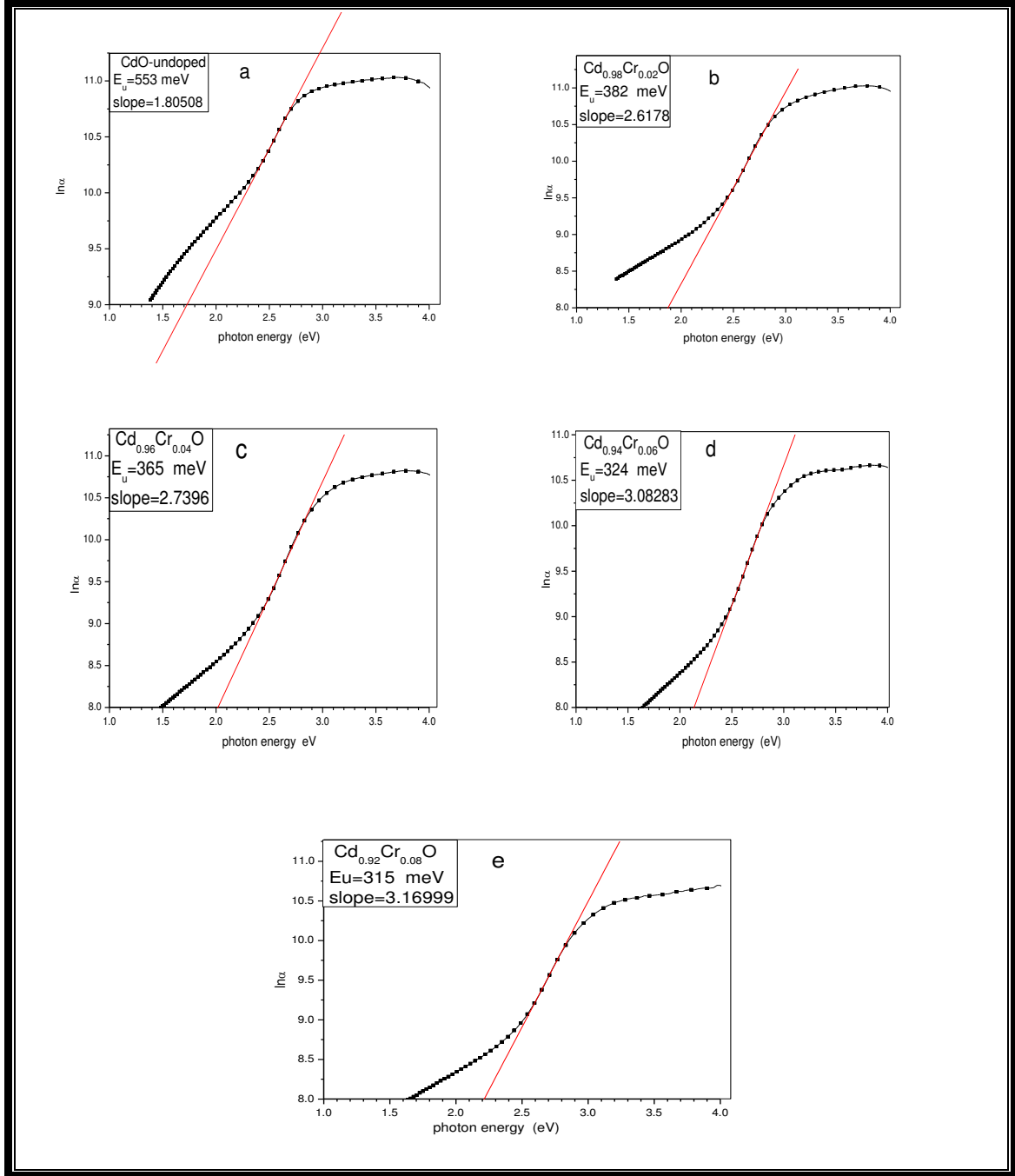
الشكل (a, b, c, d, e) قيم طاقة اورياخ لاغشية (CdO) غير المطعمة
