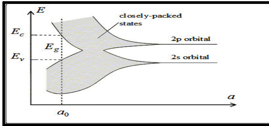
الشكل (8-2) تكون فجوة الطاقة المحظورة في المواد البلورية [62].
