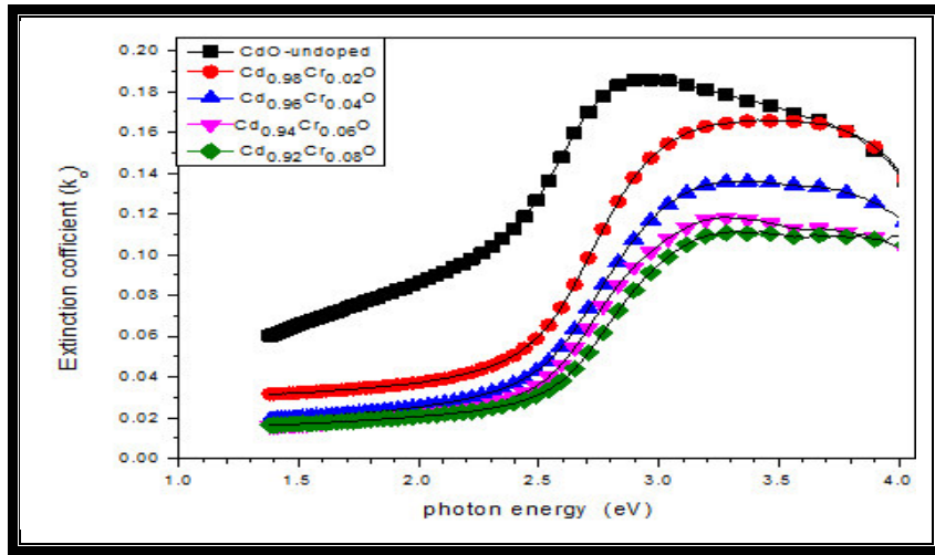
الشكل (4-18) تغير معامل الخمود كدالة لطاقة الفوتون لأغشية (CdO) غير المطعمة والمطعمة بالكروم.
