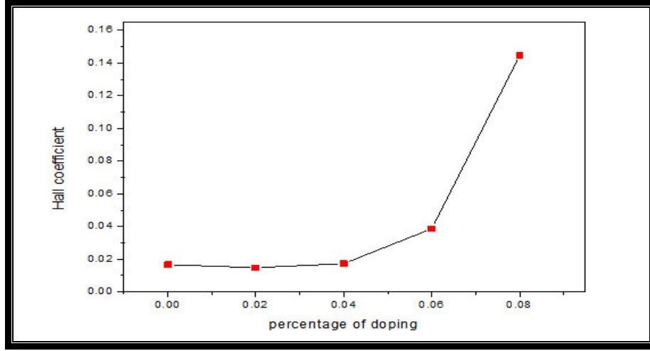
الشكل(4-26) تغير معامل هول كدالة لنسب التطعيم لاغشية (CdO) غير المطعمة والمطعمة بالكروم.
