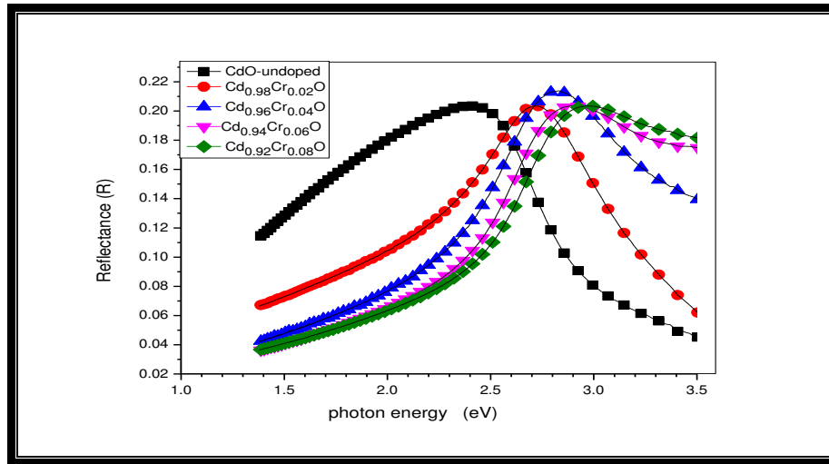
الشكل (17-4) طيف الانعكاسية كدالة لطاقة الفوتون لأغشية (CdO) غير المطعمة والمطعمة بالكروم.
