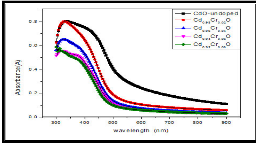
الشكل (9-4) طيف الامتصاصية كدالة للطول الموجي لأغشية (CdO) غير المطعمة
