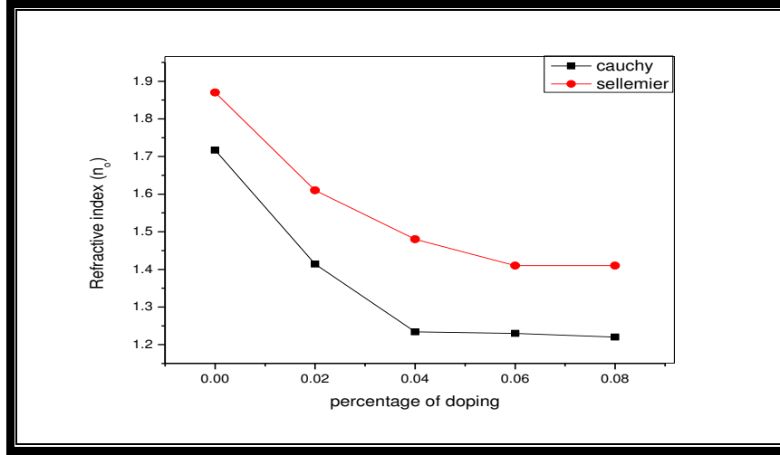
الشكل (4-22) تغير معامل الانكسار كدالة لنسب التطعيم.
