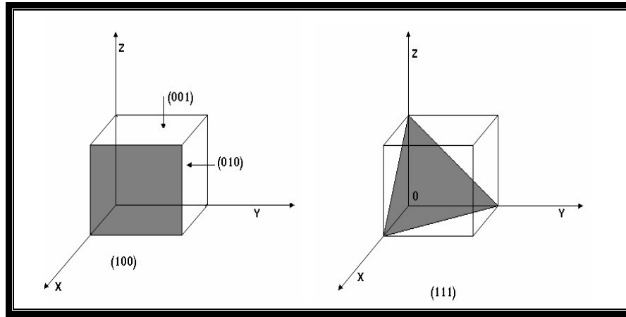
الشكل (3-2) عدد من المستويات البلورية لبلورة مكعبة [45].
