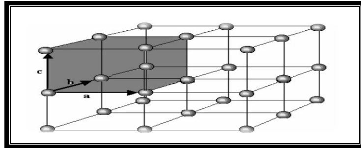
الشكل (1-2) نظام بلوري مجسم فيه وحدة خلية معينة [44].
