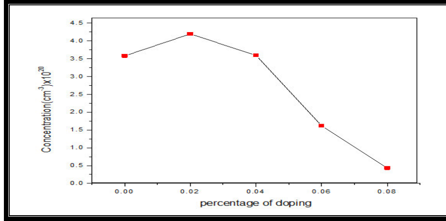
الشكل (27-4) تغير تركيز الحاملات مع نسب التطعيم لاغشية (CdO) غير المطعمة
