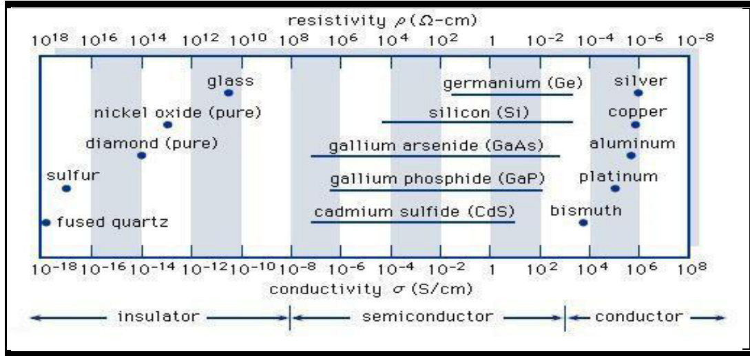
الشكل (6-2) مدى التوصيلية والمقاومية للمواد العازلة والموصلة وشبه الموصلة [59].
