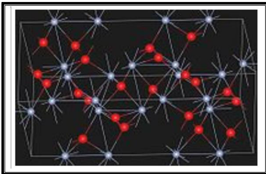
الشكل (1-8) التركيب البلوري لأكسيد الكروم [20].
