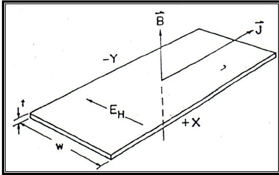
الشكل (22-2) التكوين الاساس لظاهرة هول [64].
