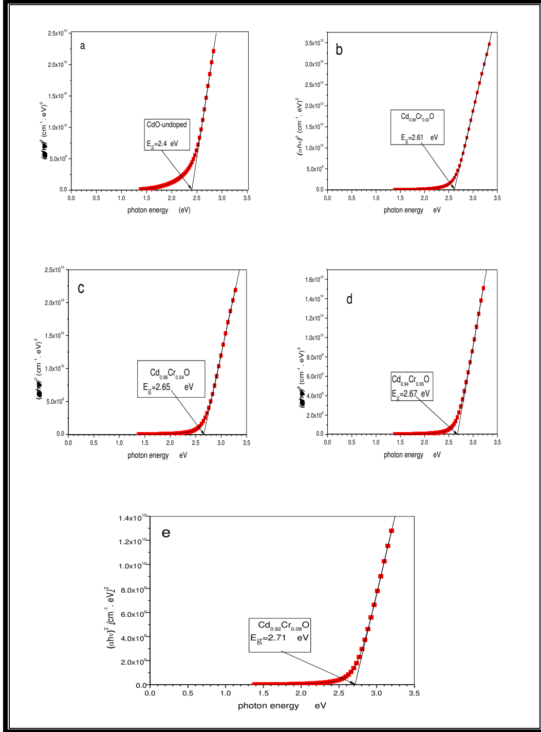
الشكل (11-4 a,b,c,d,e) قيم فجوة الطاقة كدالة لطاقة الفوتون لاغشية (CdO) غير المطعمة والمطعمة بالكروم باستعمال طريقة (Tauc).
