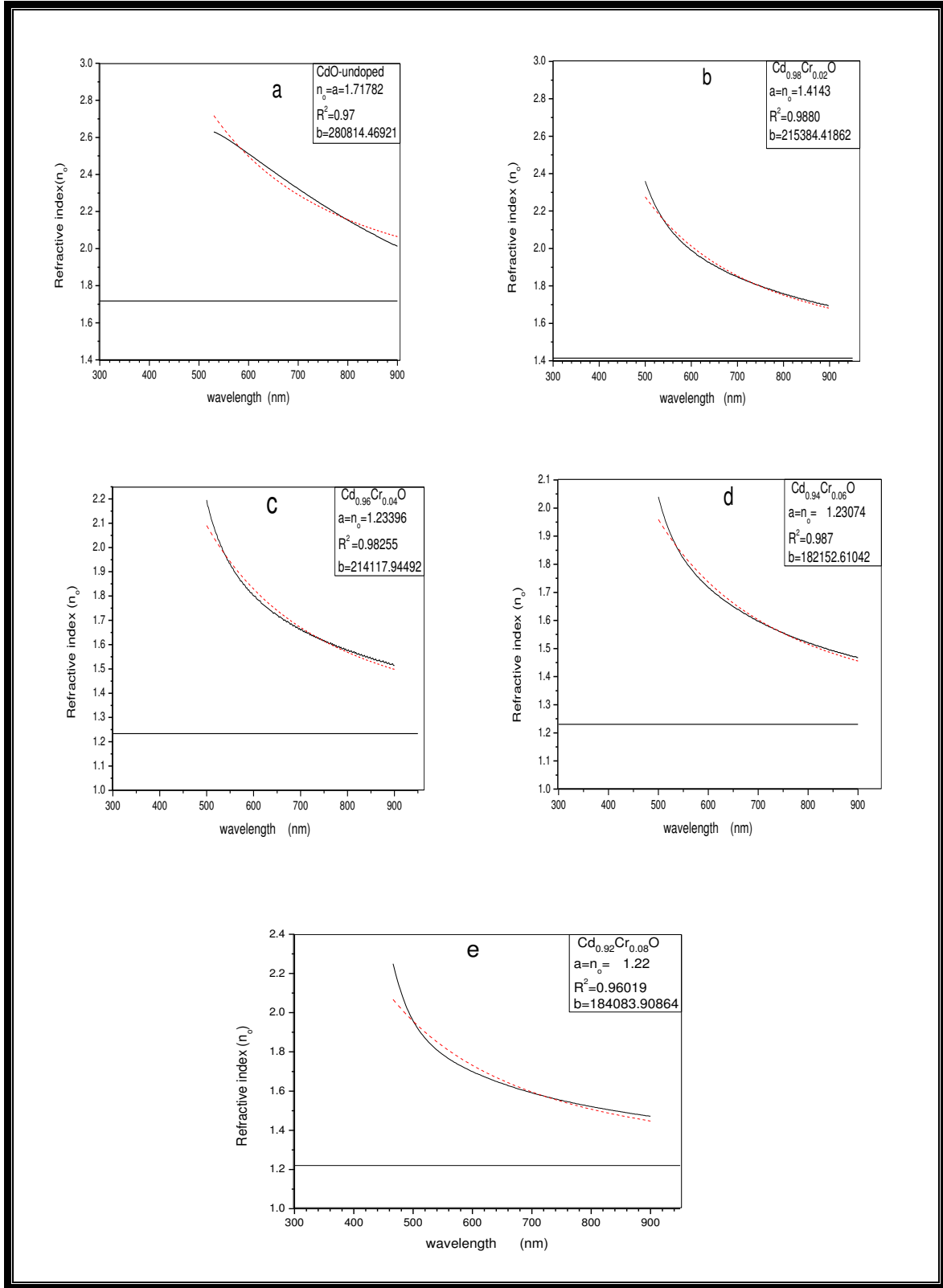
الشكل (20-4 a,b,c,d,e) العلاقة بين معامل الانكسار والطول الموجي (نموذج Cauchy)
