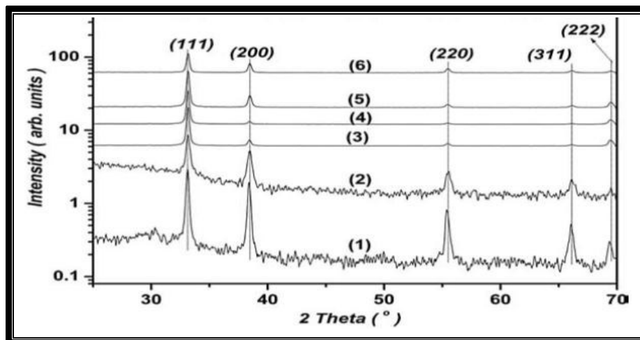
الشكل (2-12) انماط حيود الاشعة السينية لأغشية أكسيد الكاديوم غير المطعمة والمطعمة بالحديد [29].
