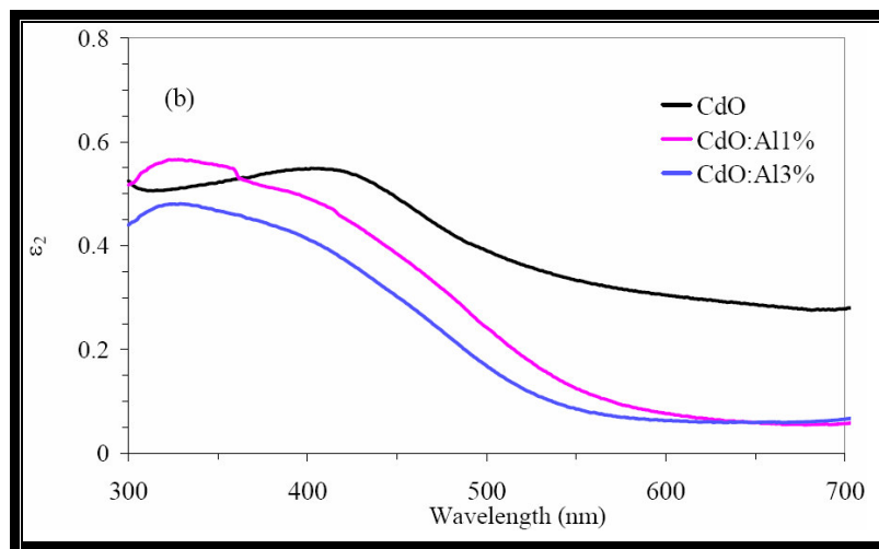
الشكل (21-2) تغير ( \epsilon_2 ) مع ( \lambda ) لأغشية (CdO) غير المطعمة
