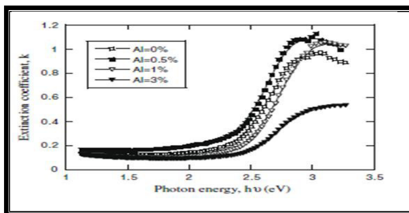
الشكل (18-2) معامل الخمود كدالة لطاقة الفوتون لآغشية (CdO:Al) [30].
