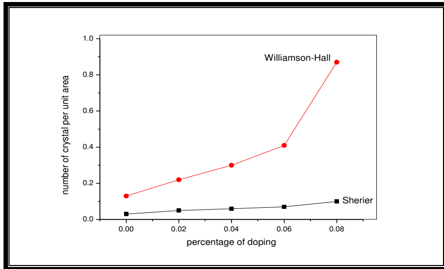
الشكل (5-4) قيم عدد البلوريات لوحدة المساحة كدالة لنسب التشويب.
