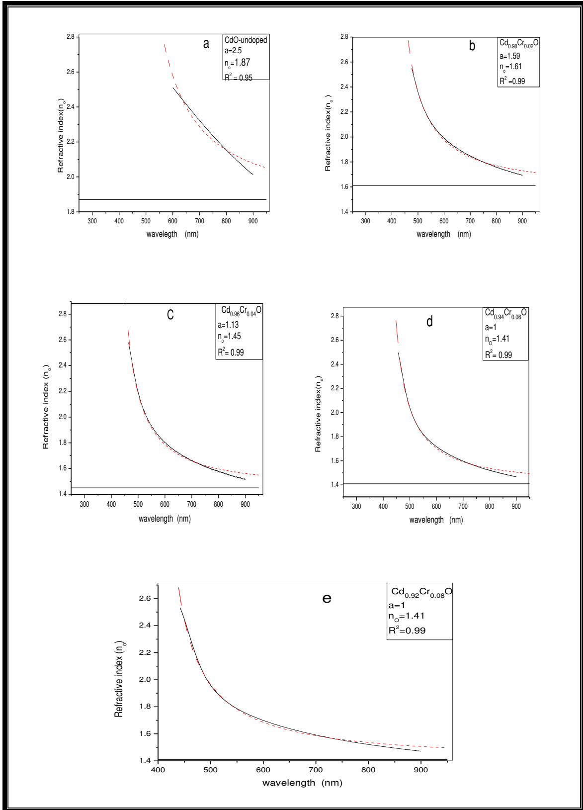
الشكل (21-4 a,b,c,d,e) العلاقة بين معامل الانكسار والطول الموجي لاغشية (CdO) غير المطعمة والمطعمة بالكروم انموذج (Sellmeier).
