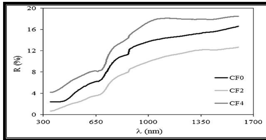
الشكل (17-2) الانعكاسية كدالة للطول الموجي لآغشية (CdO) المطعمة بالفلور [78].
