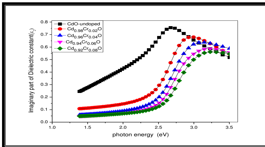
الشكل (24-4) تغير ثابت العزل الخيالي كدالة لطاقة الفوتون لأغشية (CdO) غير المطعمة والمطعمة بالكروم.
