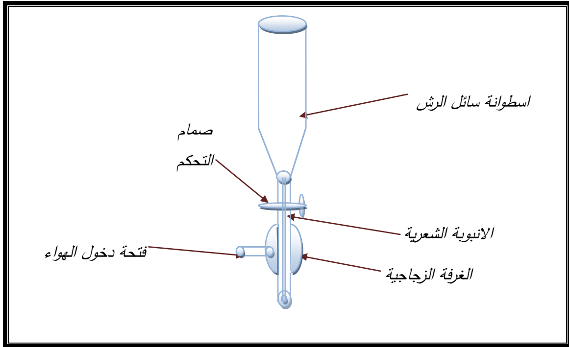
الشكل (3-3) اجزاء جهاز التبريد
